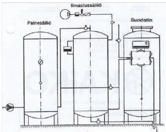
JK-LH & LK suodattimien kytkentäkaavio
