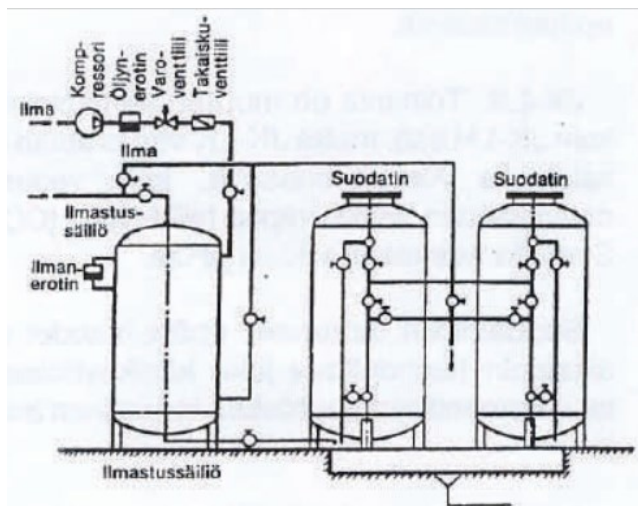
JK-LH & LK laitteiston kytkentäkaavio, kun suodattimia on kaksi rinnan.
